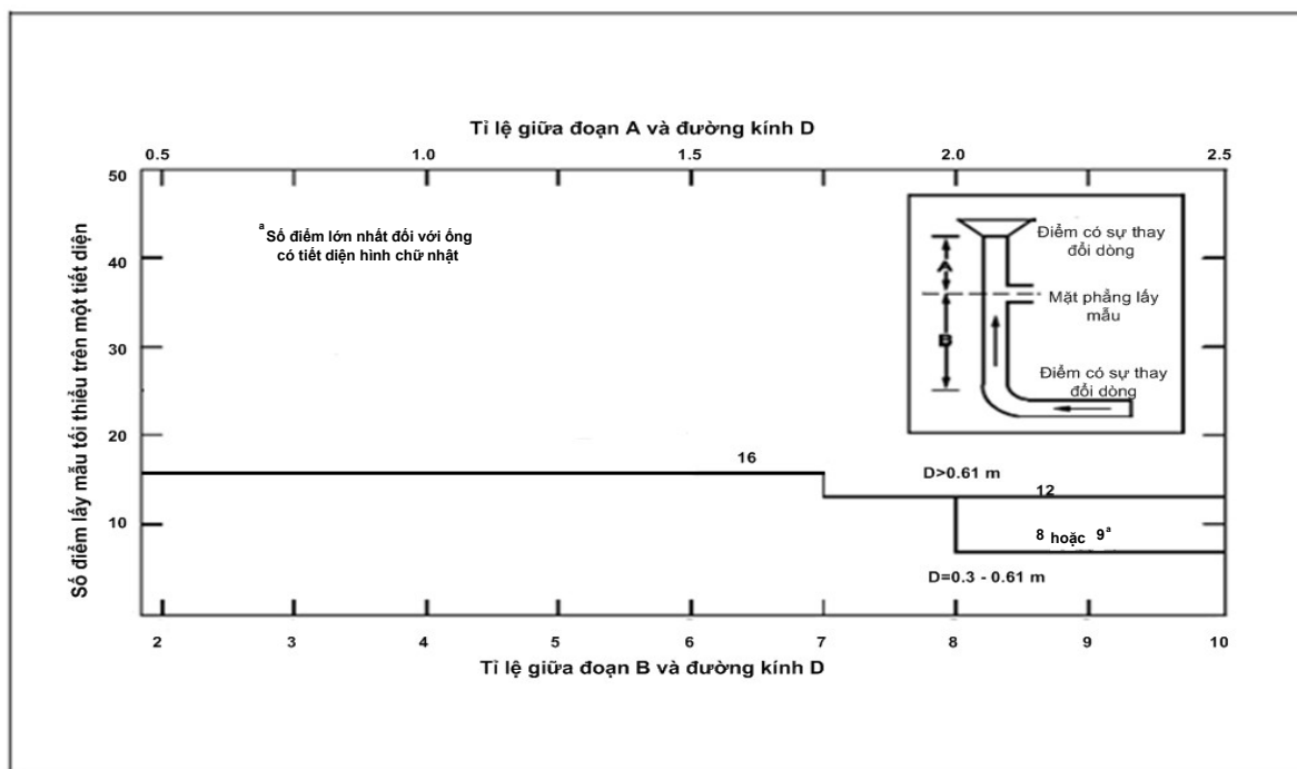
Hình 2. Đồ thị lựa chọn số điểm hút mẫu tối thiểu theo phương ngang (chỉ xác định vận tốc)
